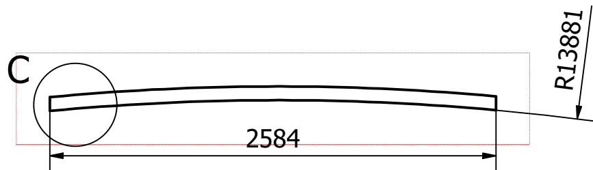
CHI TIẾT 5:Thép hộp 80x40x5 - SL: 2 - TL: 1:10
