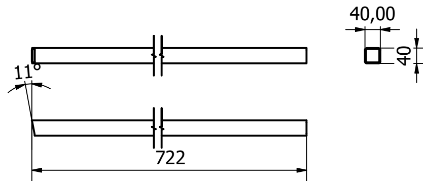
CHI TIẾT 8:Thép hộp 40x40x2.5 - SL: 2 - TL: 1:10
