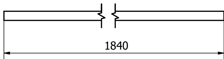
CHI TIẾT 5:Thép hộp 80x40x5 - SL: 2 - TL: 1:10
